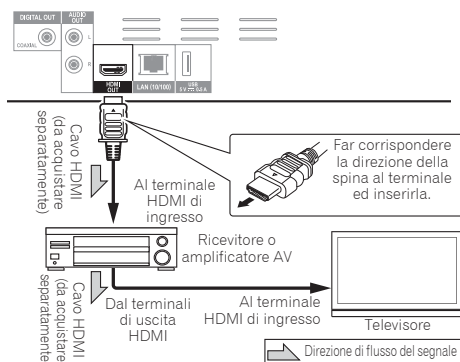
Pannello posteriore
